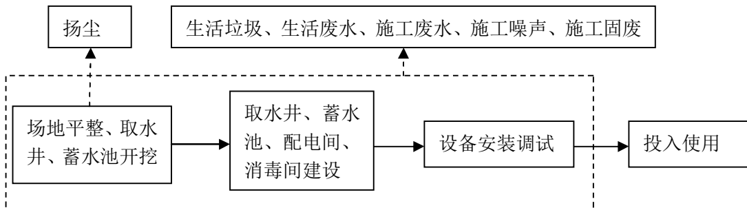
图 2 取水井、配电间、加氯间-配电间、蓄水池施工工艺及产污环节图
