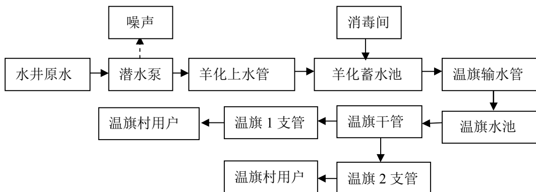
图 4 运营期工艺流程及产污节点图
