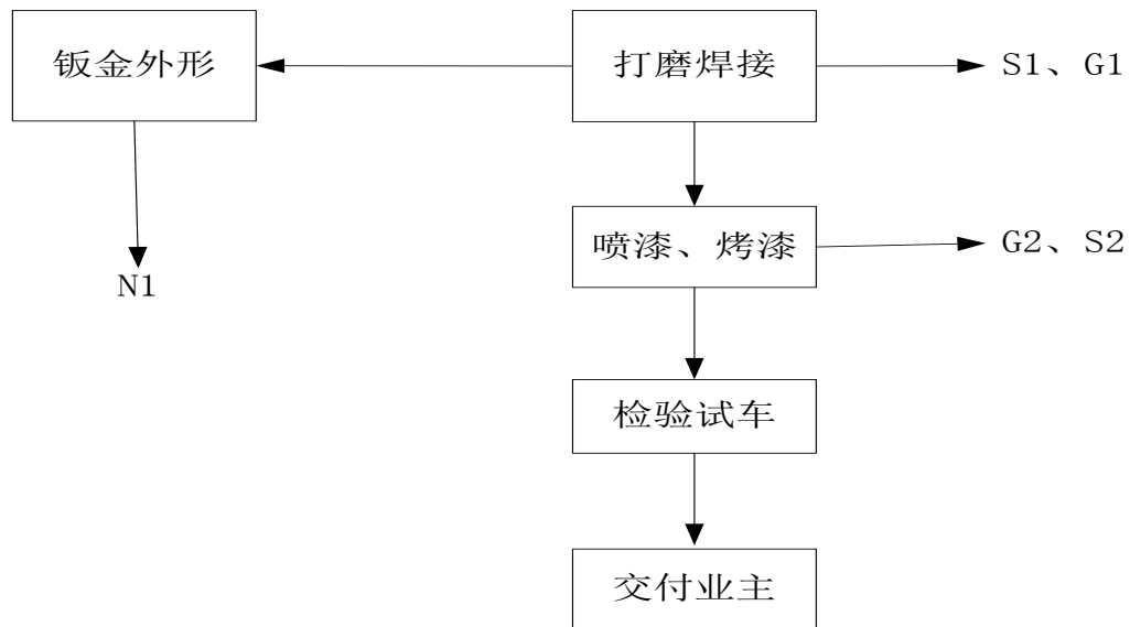
图3 钣金喷漆工艺流程及产污节点示意图
