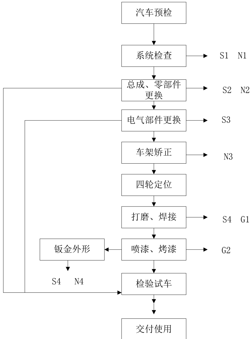
图2 专业保养维修服务工艺流程及产污节点示意图
