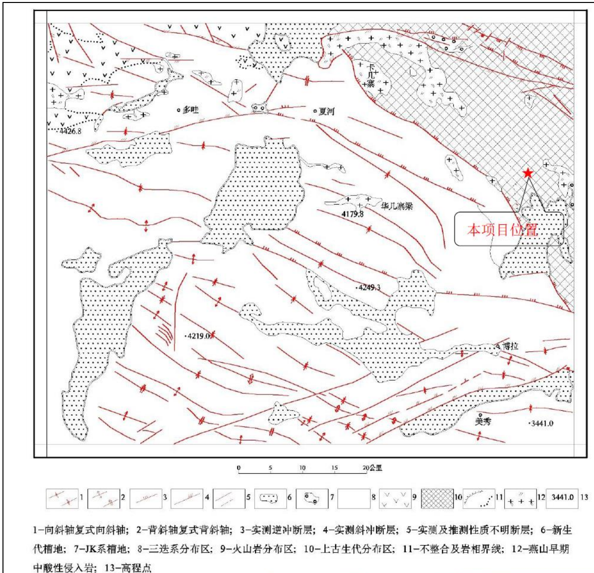
图 4 评价区地质构造图
