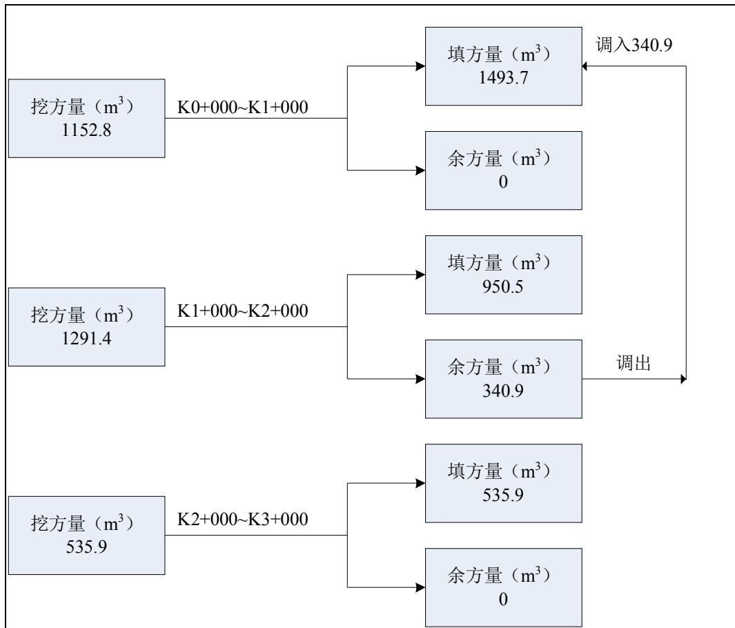
图 2-4 项目土石方平衡图 单位：m 3
