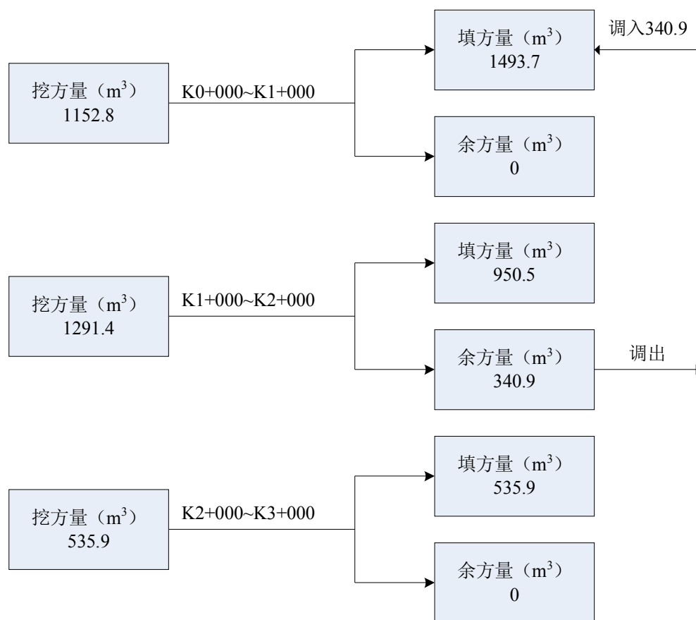
图 2 项目土石方平衡图
