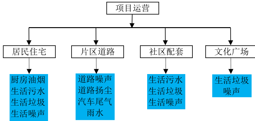
图 11 运营期产污节点示意图
