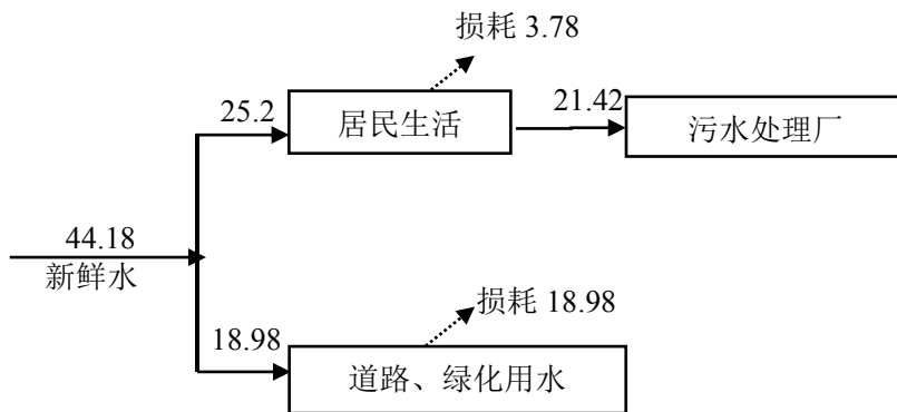
图 9 日用水平衡图（单位：m 3 /d）
