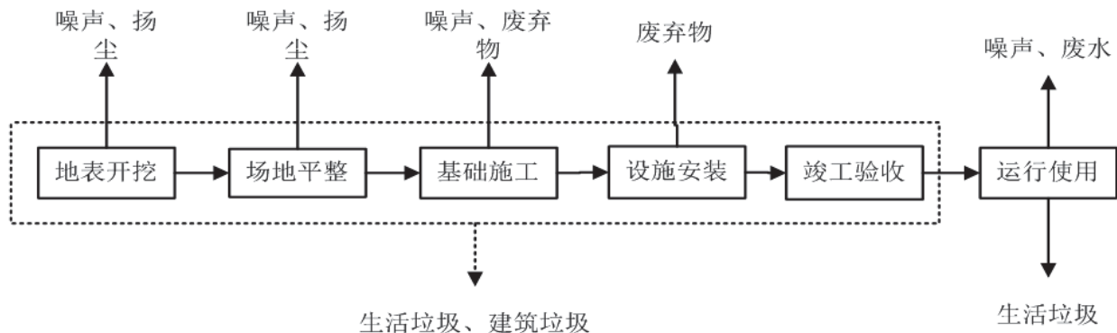
图 5-1 项目施工期、运行期工艺流程及排污节点图
