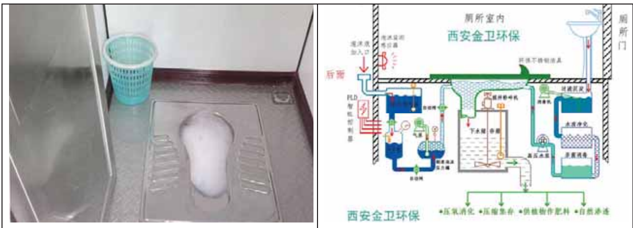
免冲泡沫式环保厕所效果图
