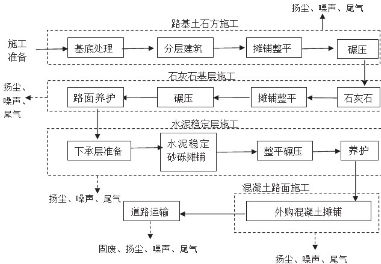
图 5-2 道路施工工艺流程及产污节点图
