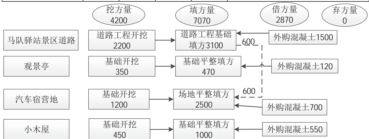
图 5-2 项目土石方平衡示意图 单位： m^3
