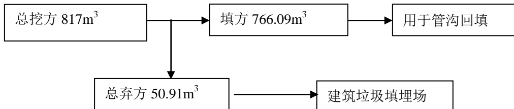
图 3 项目土石方平衡表
