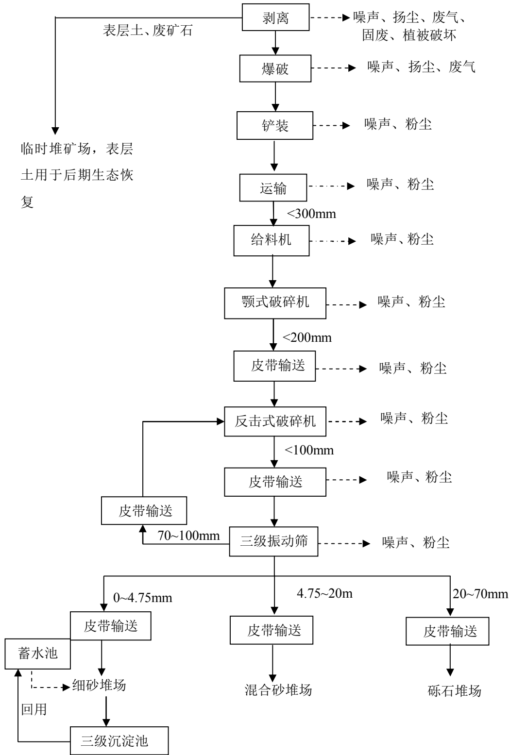
图 2.4-1 项目生产工艺流程及产污位置图
